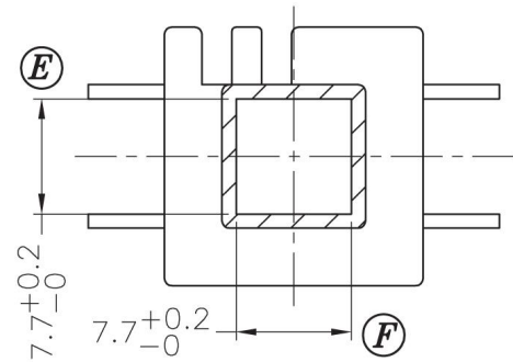
SEC.A-A
