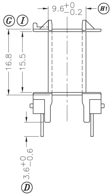
SEC.A-A
